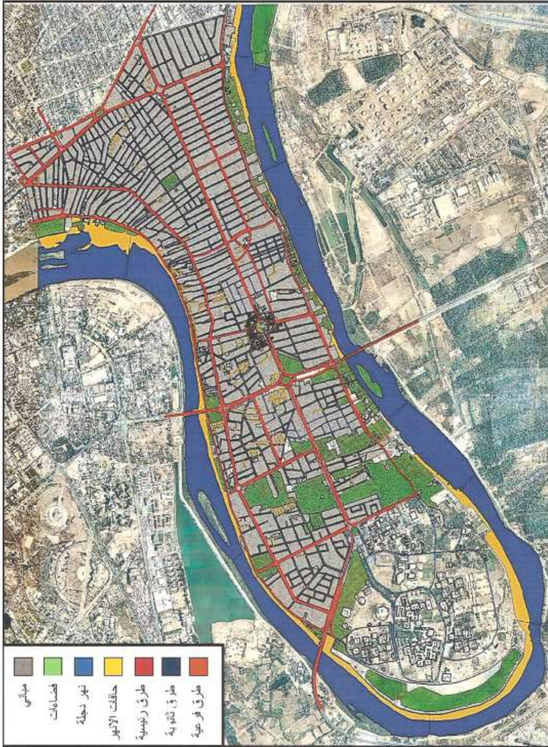
الشكل (٣) : يوضح واقع الحال للمباني والفضاءات والحركة لمنطقة الكرادة / إعداد الباحث
